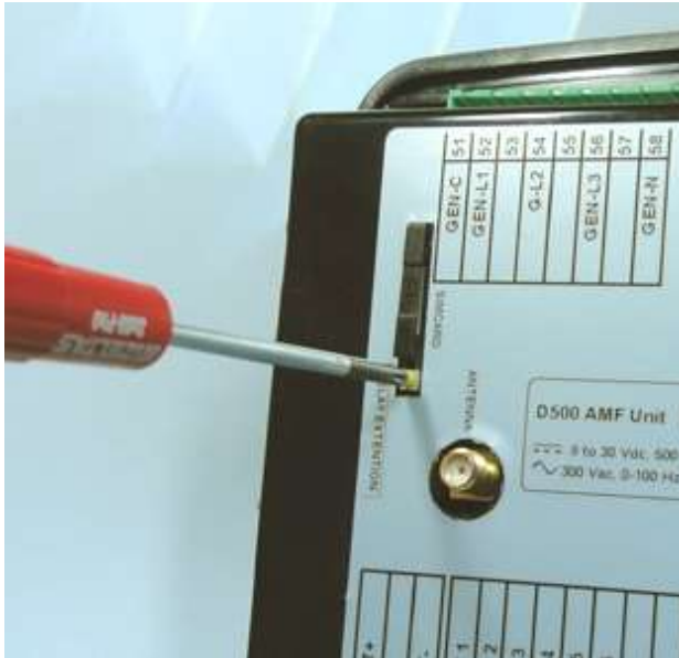
Извлечение SIM карты
